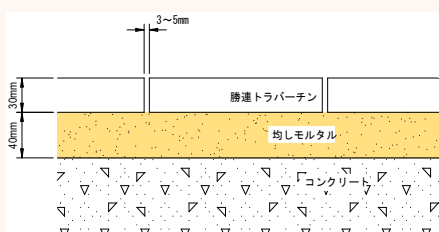
標準断面
